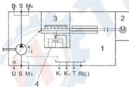
EM Schematic
